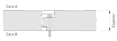
Detalle sistema fijación
