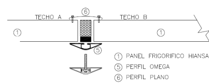
SUSPENSIÓN TECHO POR OMEGA
