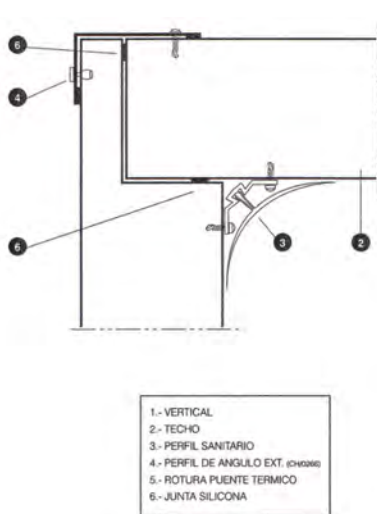
ENTREGA PANEL CONSERVACIÓN
