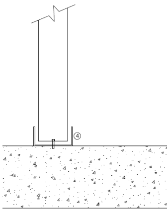
ARRANQUE PANEL CONSERVACIÓN
