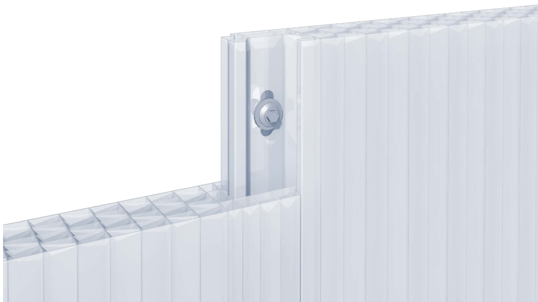
DETALLE ENTREGA ENTRE PLACAS DE POLICARBONATO EN CONTÍNUO
