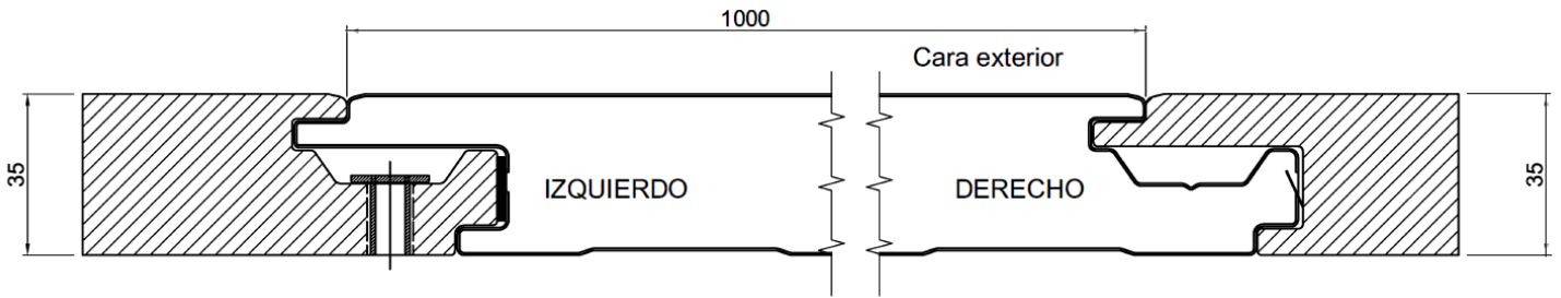
DETALLE ENTREGA POLICARBONATO - PANEL FACHADA - FIJACIÓN OCULTA
