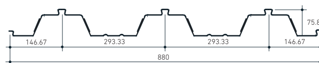
SECCIÓN PERFIL
