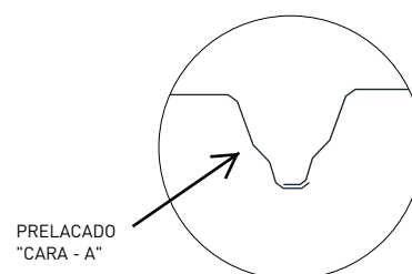
DETALLE SOLAPE
